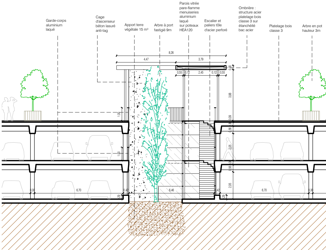
Coupe d'une trémie et d'un édicule d'accès au parking
