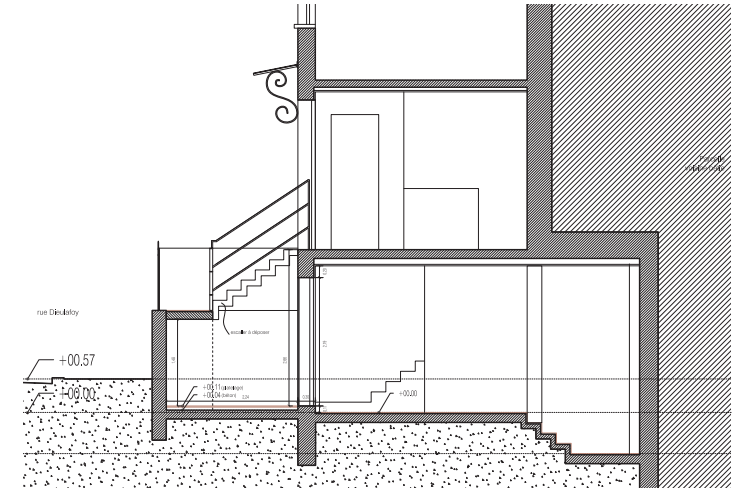
Élévation sur rue et coupe de l'existant
