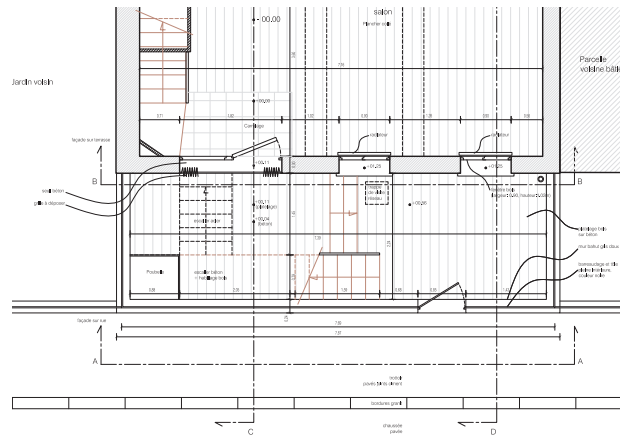
Plan de l'accès existant depuis la rue : grille et portillon, volées d'escaliers dans la courette, accès décalé au salon
